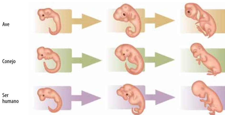
Semejanzas en el desarrollo embrionario de vertebrados.
