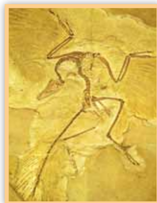
Resto fósil de un Archaeopteryx .
