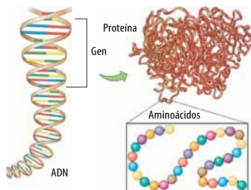
Estructura de una molécula de ADN y una proteína.
